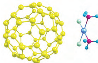
Рис. 3. Розрахована оптимальна структура наноконкомпозиту C_{60} -фулерену із цисплатиною
