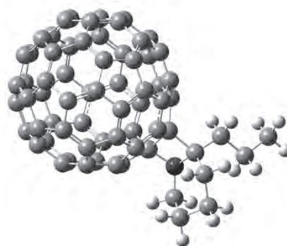
Рис. 1. Розрахована оптимальна структура наноконкомпозита на основі алкалоїду \gamma -коніциїну та C_{60} -фулерену [9]
