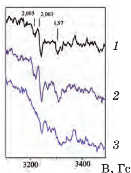
Рис. 4. Спектри ЕПР ДР: офіційний ДР (1), ММХА з використанням сталевих (2) та агатових (3) кульок
