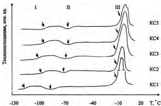
Рис. 1. Термограммы многокомпонентных криозащитных сред при нагреве от T = -196\text{ }^{\circ}\text{C} (пояснения в тексте)
