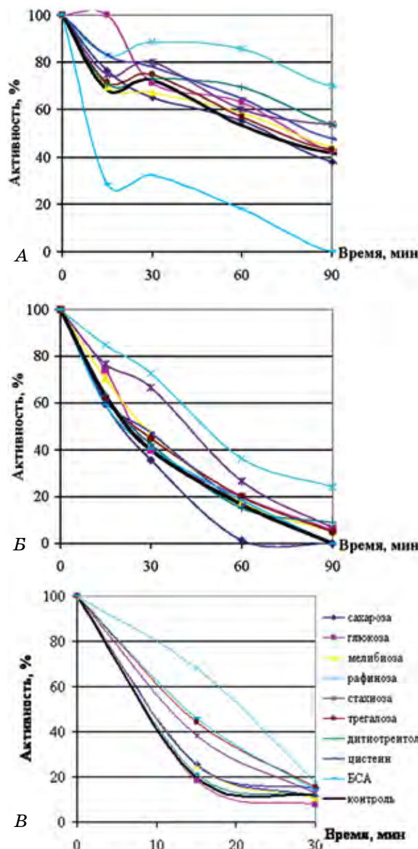
Рис. 4. Кинетические кривые термоинактивации \alpha -галактозидазы A. niger при 51 °C (А), 54 °C (В), 57 °C (В) в присутствии различных веществ
