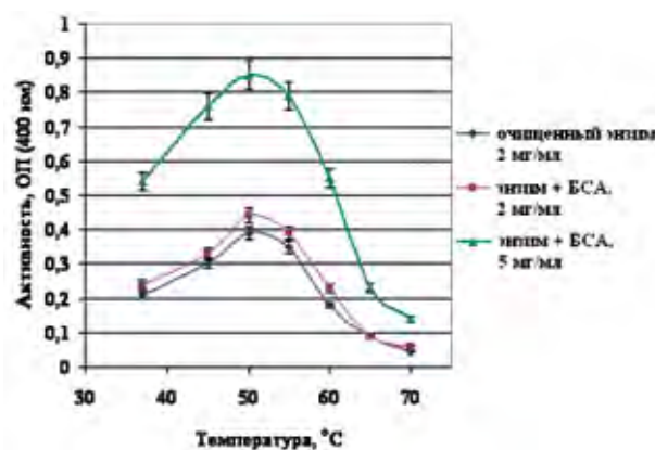
Рис. 1. Термооптимум \alpha -галактозидазы A. niger (рН 5,7)
